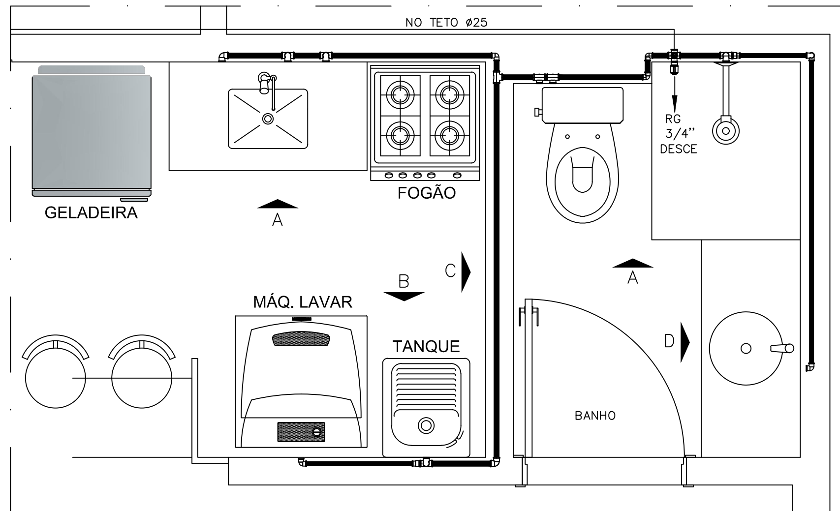
Plano de Cozinha e Banheiro para os apartamentos 304 a 1504 e 411 a 1511. ESCALA 1/25
